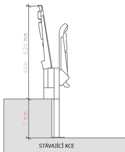
BOČNÍ POHLED
