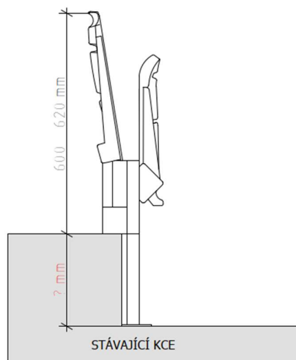
BOČNÍ POHLED
