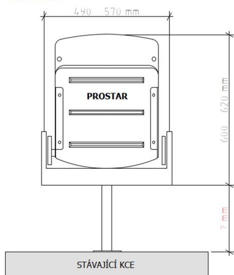
ČELNÍ POHLED
