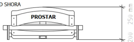
POHLED SHORA
