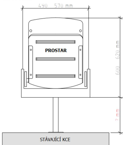
ČELNÍ POHLED
