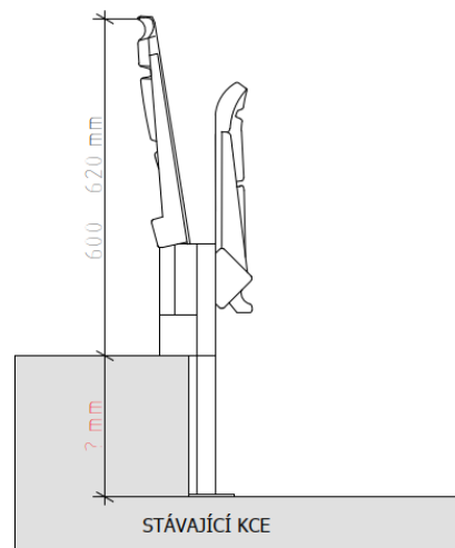
BOČNÍ POHLED
